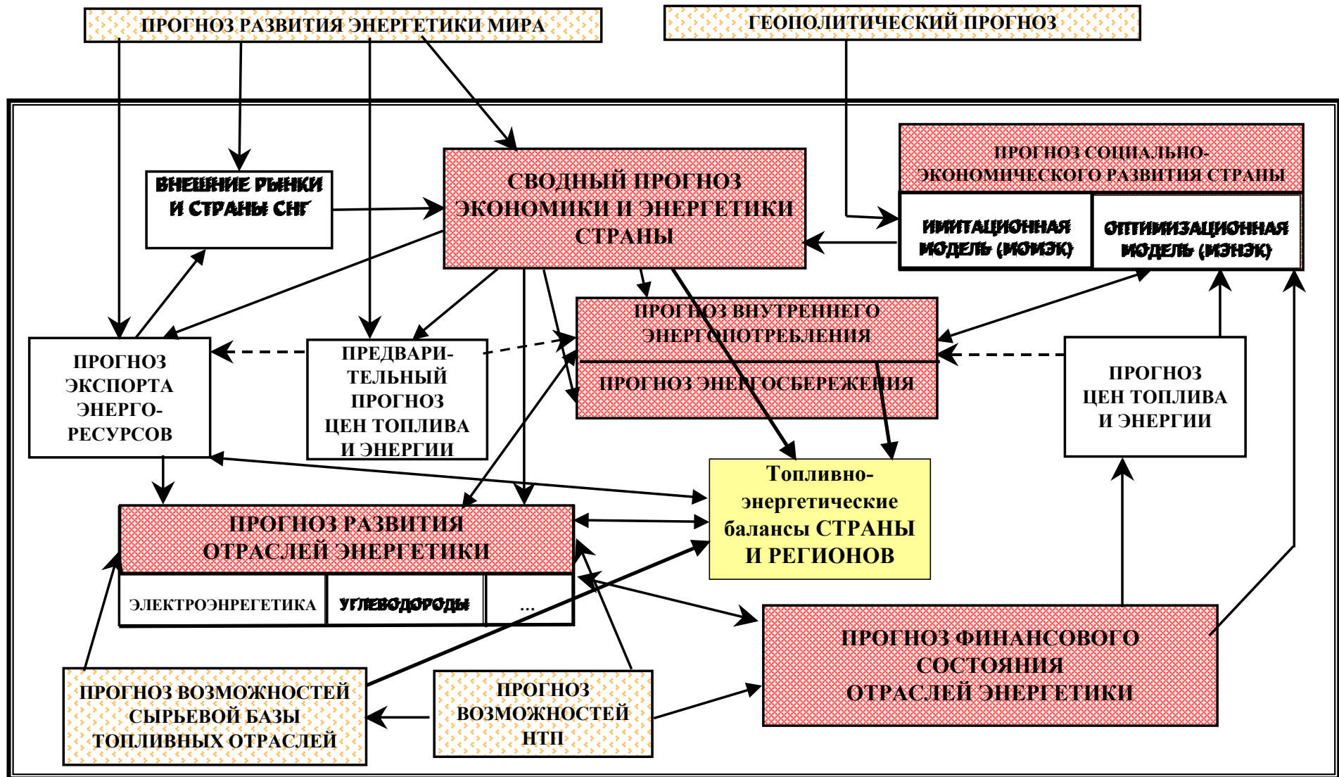
Рис. 4П. Общая схема прогнозирования энергетики России
